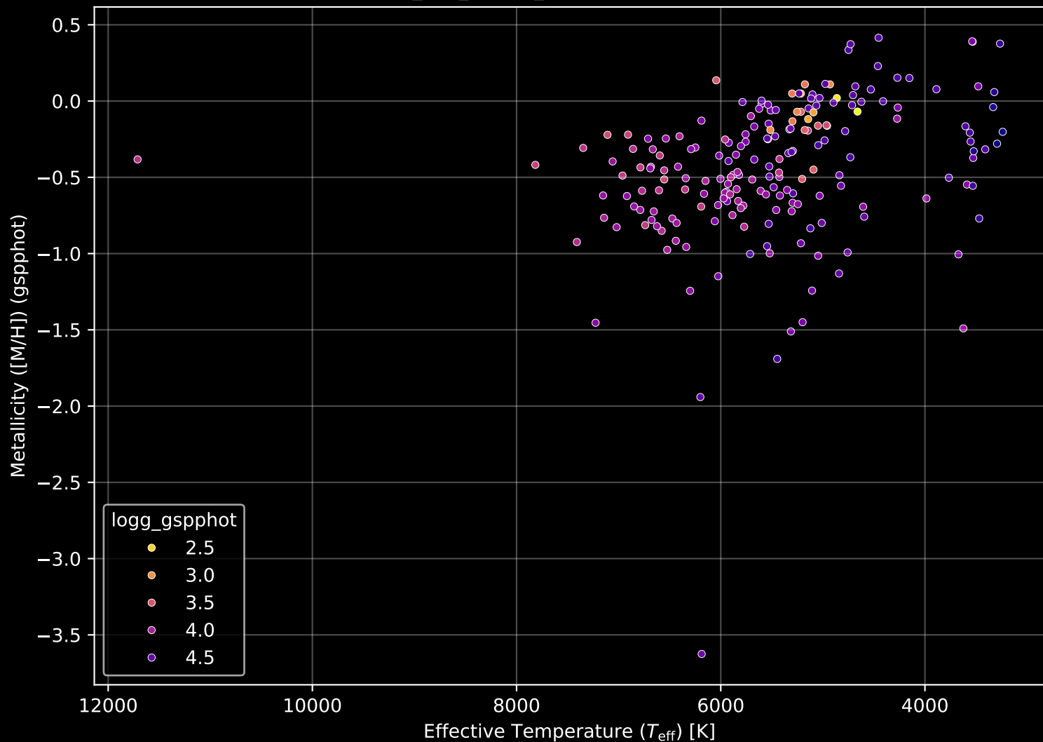
APOGEE DR17 Field: [K2_C13_181-21_btx] Stellar Population Parameters (n= 200)
